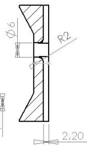
SECCIÓN D-D
